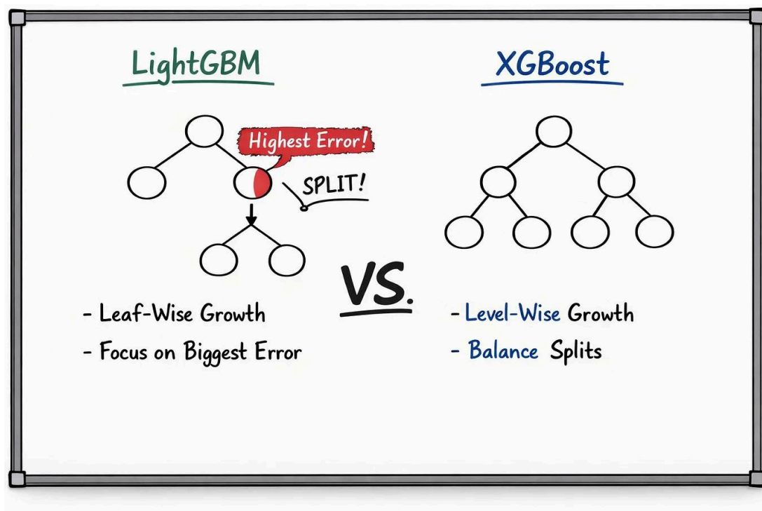
Hình 1.5. Thuật toán LightGBM
