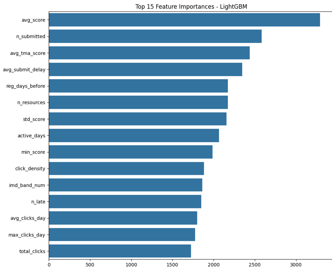
Hình 3.10. Biểu đồ top feature importances với mô hình học máy
