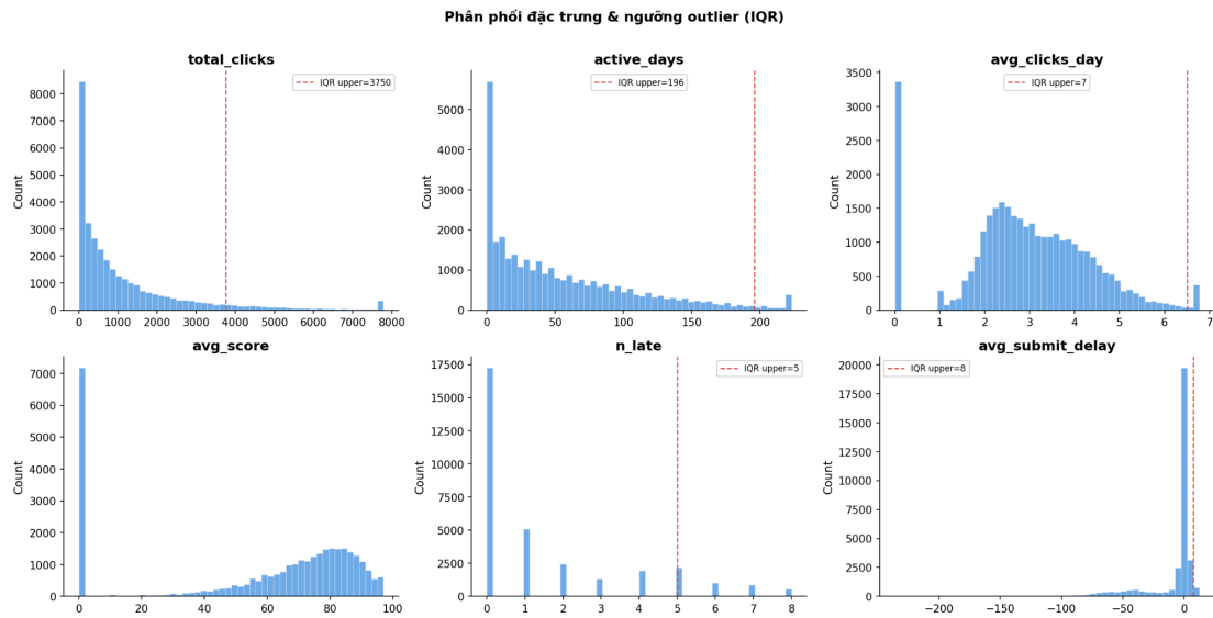
Hình 3.6. Biểu đồ hiển thị các biến outlier làm lệch giá trị trung vị và ngưỡng.
