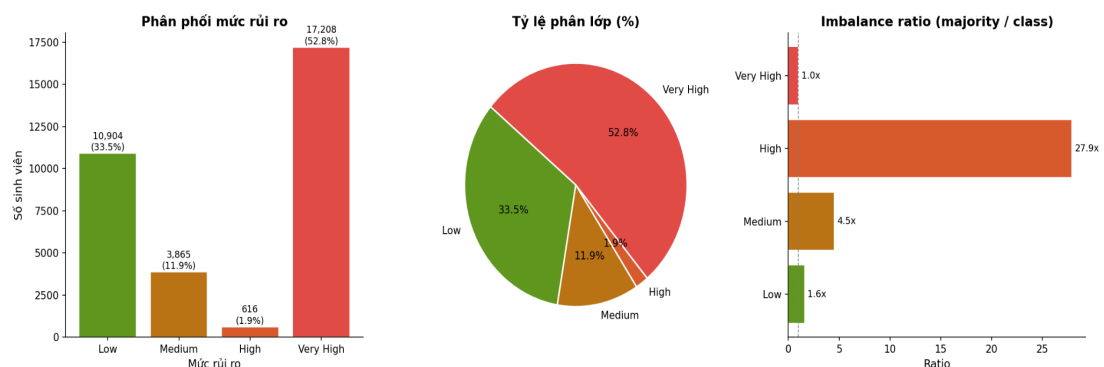
Hình 3.7. Biểu đồ trực quan hóa dữ liệu mất cân bằng giữa các lớp phân loại rủi ro.
