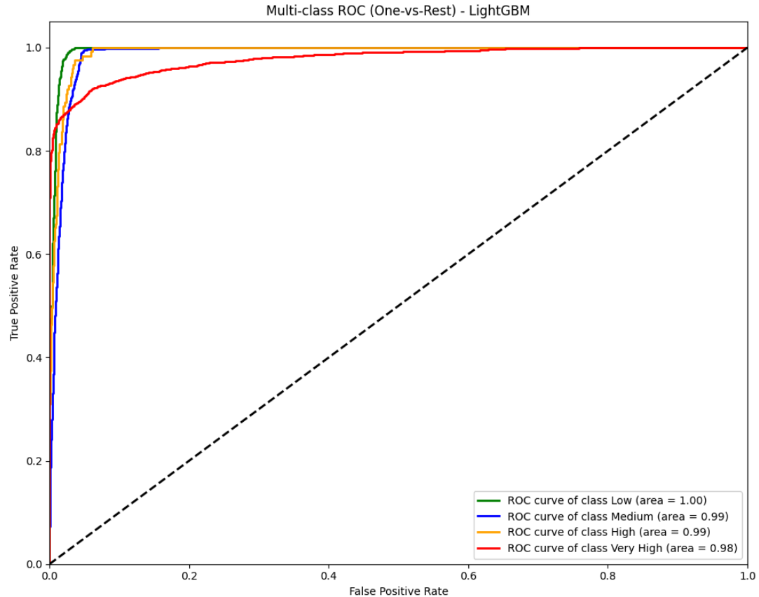
Hình 3.9. Biểu đồ đánh giá ROC Curve trên từng nhãn rủi ro bằng mô hình LightGBM.
