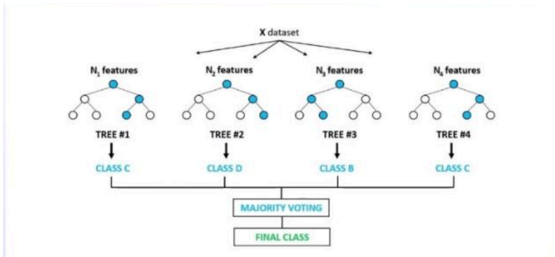
Hình 1.3. Máy học Random Forest
