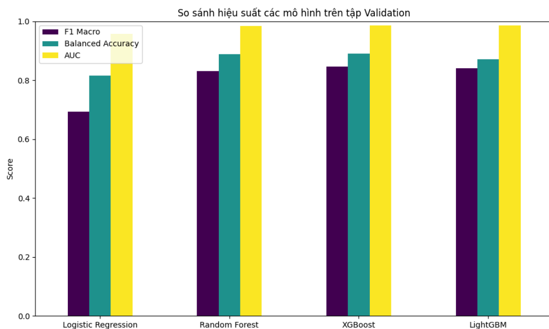
Hình 3.8. Biểu đồ so sánh thông số AUC, F1-Score và Balanced Accuracy giữa các thuật toán Machine Learning.
